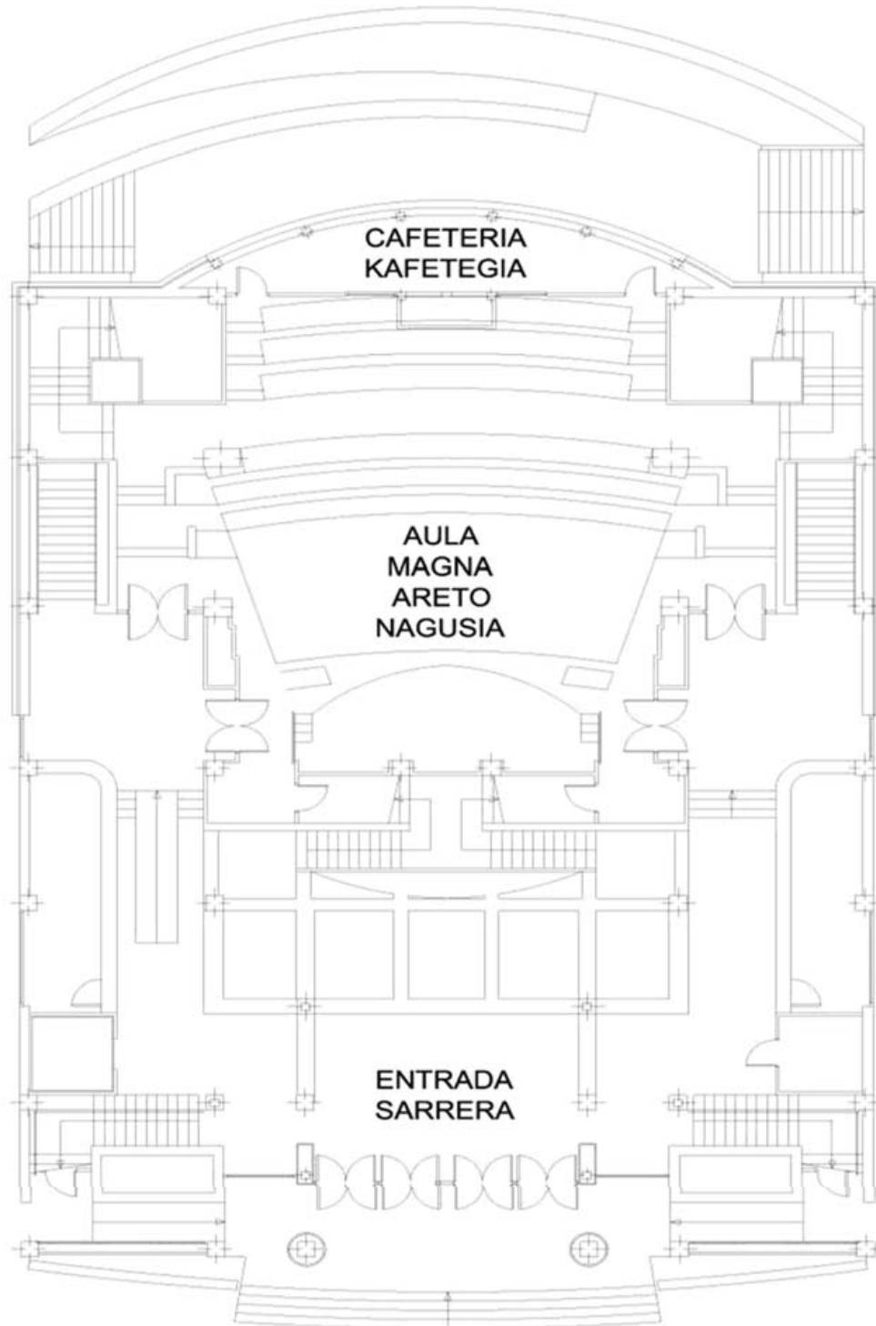
PARTE CENTRAL PLANTA BAJA ERDIGUNEKO BEHEKO SOLAIRUA
